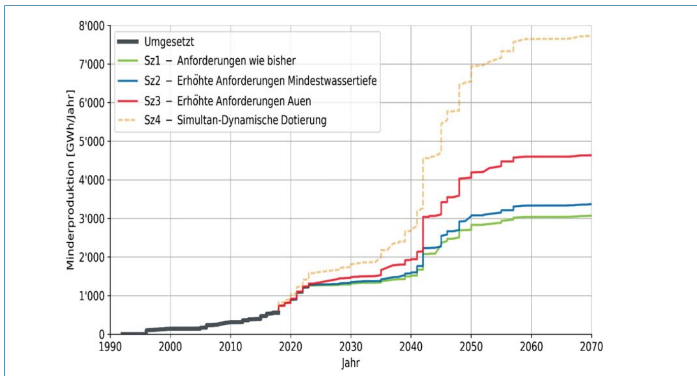
Bild 4. Summenkurven der ermittelten Energieeinbussen je nach hinterlegtem Szenario im Zeitverlauf von 1992 bis 2070.
